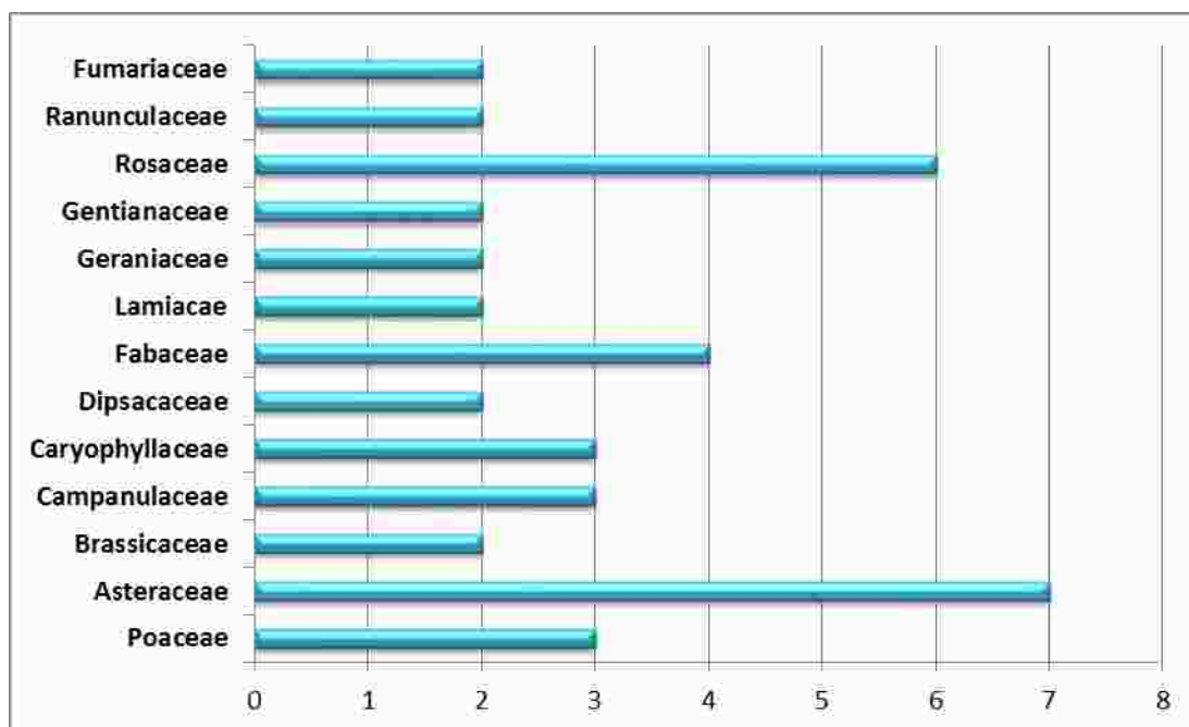
გრაფიკი 11. ენდემური სახეობების განაწილება ოჯახების მიხედვით
