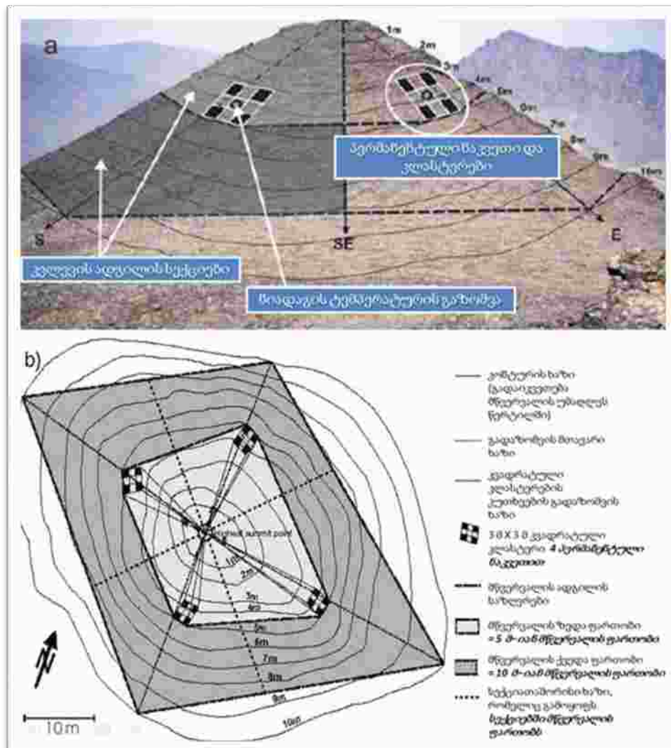
სურათი 10. მწვერვალებისა (a) და სამონიტორინგო ნაკვეთების (b) სტანდარტული სქემა
