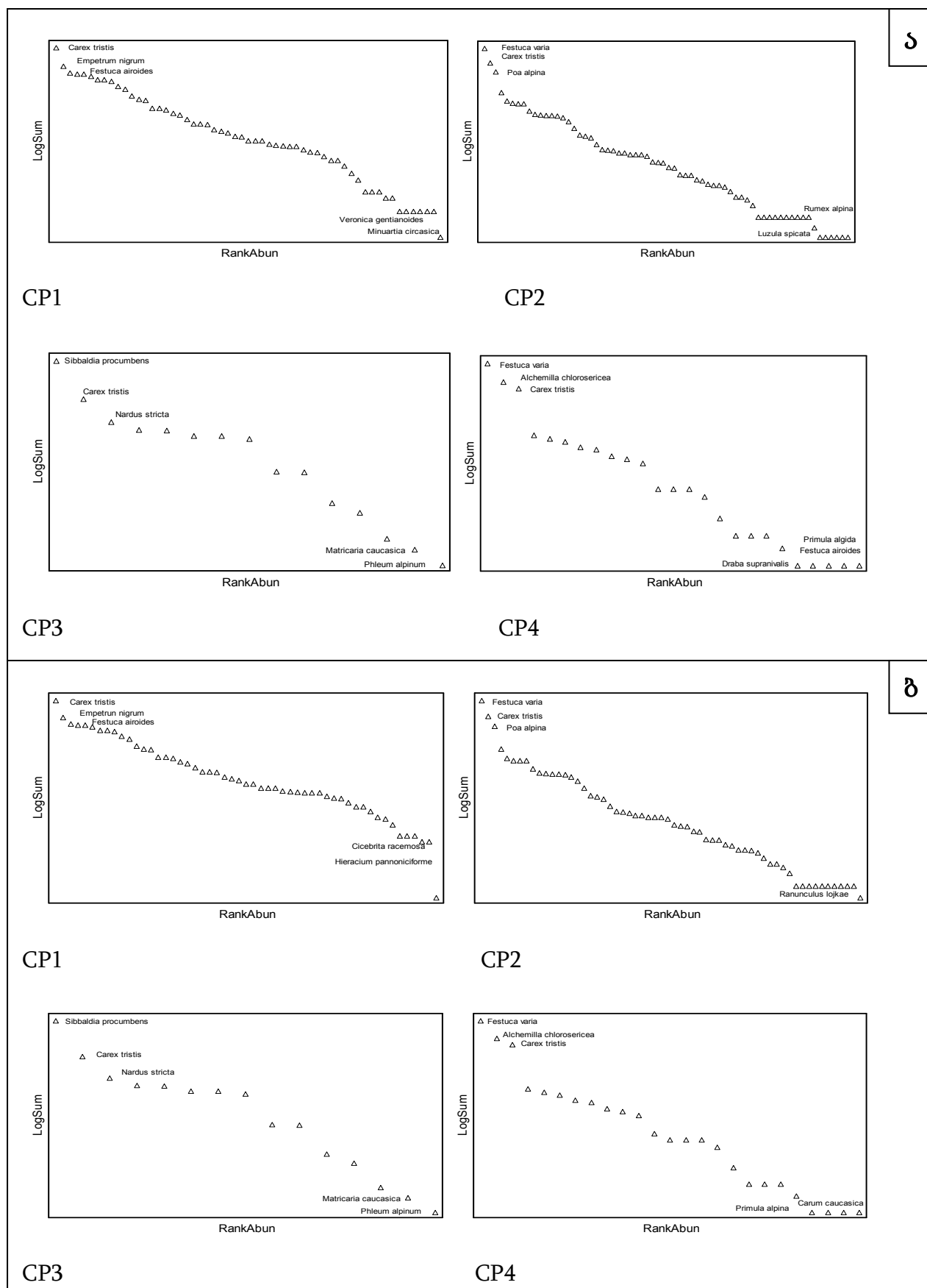
გრაფიკი 17. დაფარულობის მოხედვით დომინანტი სახეობები 2001 (ა) და 2008 (ბ) წელს (PCORD სტატისტიკური პროგრამის სახეობათა დომინანტობის ტესტი).
