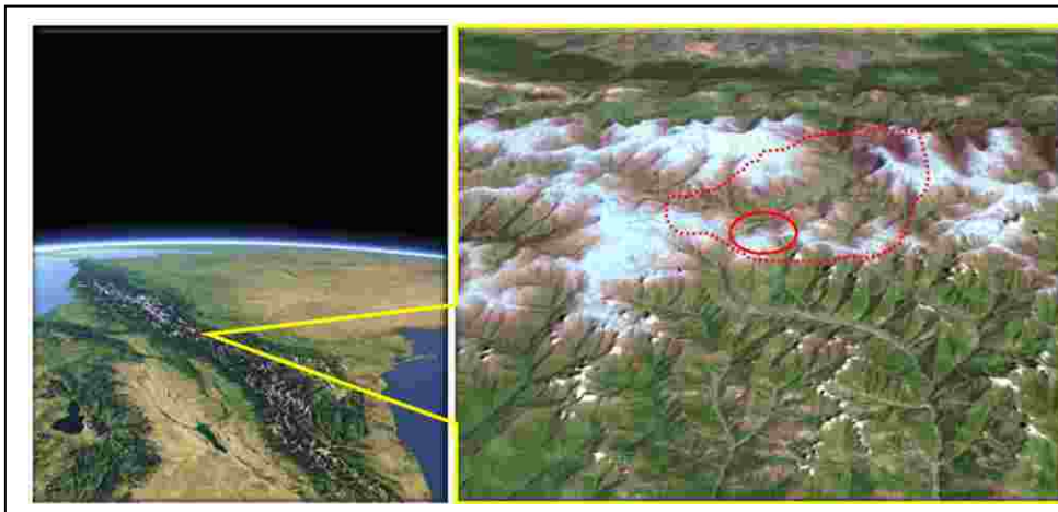
სურ. 1. კავკასია, დიდი კავკასიონი, ცენტრალური კავკასიონი, ყაზბეგის რეგიონი (პუნქტირით), გუდაურის მიდამოები (უწყვეტი ხაზით)
