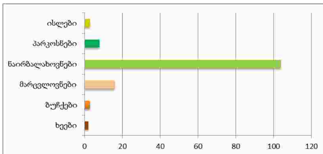
გრაფიკი 9. სამონიტორინგო ფართობებზე სახეობათა სხვადასხვა ფუნქციური ჯგუფის პროცენტული განაწილება
